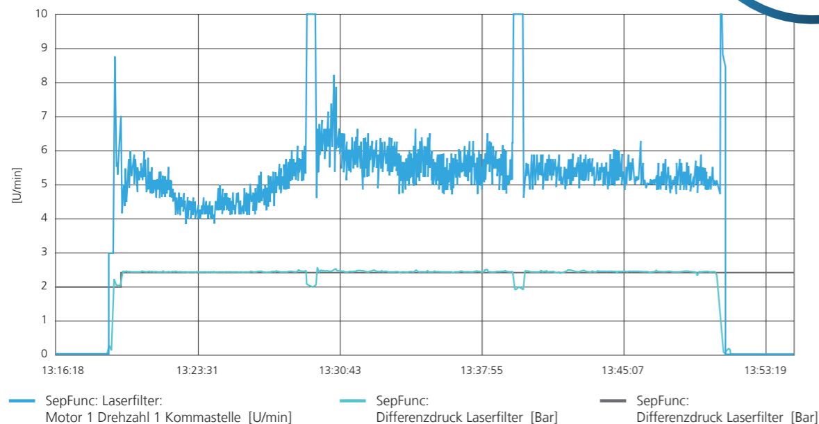
Trendverlauf Laserfiltersteuerung
